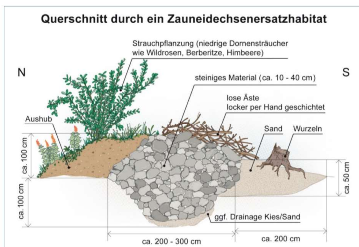
Prinzi skizze eines Ersatzhabitats Quelle: Arbeitshilfe Zauneidechse, LFU 2020
